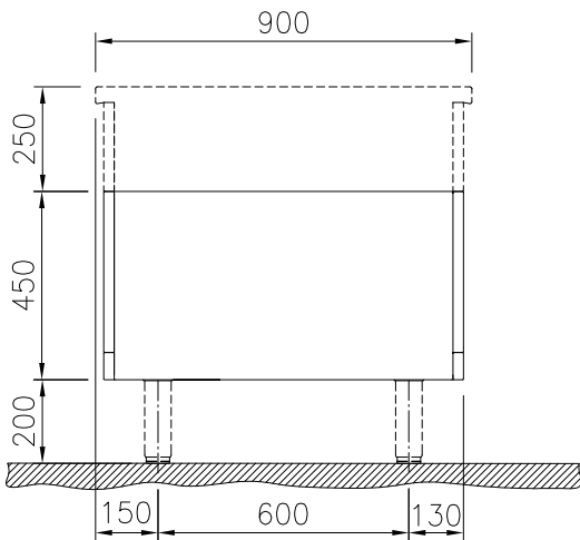
俯视
